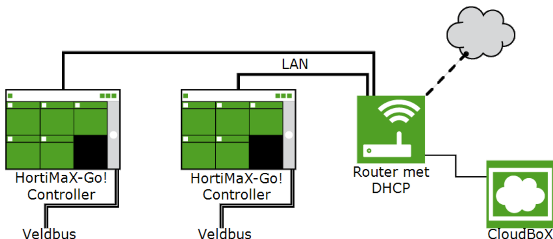
Figuur 1-1: Schematische weergave netwerkaansluiting.
